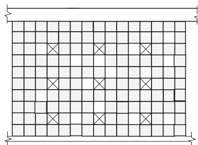
План подвесного потолка (армстронг 600x600 мм) с ориентировочным расположением светильников
